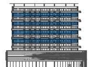
ELEVATION A
